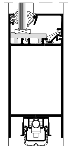
Schüco Дверь ADS 50.NI, масштаб 1:2 Schüco Door ADS 50.NI, scale 1:2
