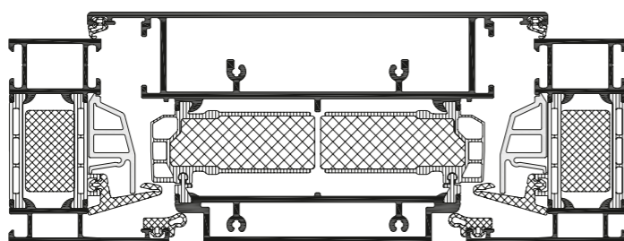
Горизонтальное сечение вентиляционной створки Schüco AWS VV Horizontal section detail of Schüco Ventilation Vent AWS VV
